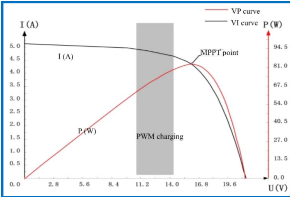
Figure 1-2 Caractéristique de la courbe de sortie du panneau solaire
