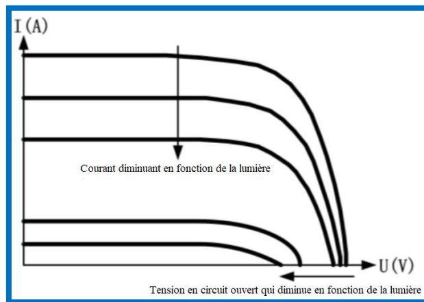
Figure 1-3 Relation entre les caractéristiques en sortie du panneau solaire
