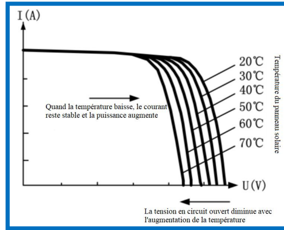
Figure 1-4 Relation entre les caractéristiques de sortie du panneau solaire et la température
