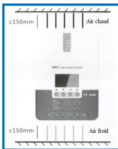
Figure 2-1 Installation et dissipation de chaleur
