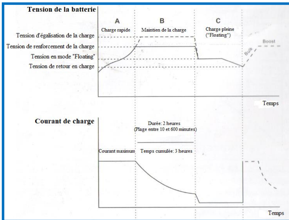
Figure 1-5 Diagramme d'état de charge d'une batterie
